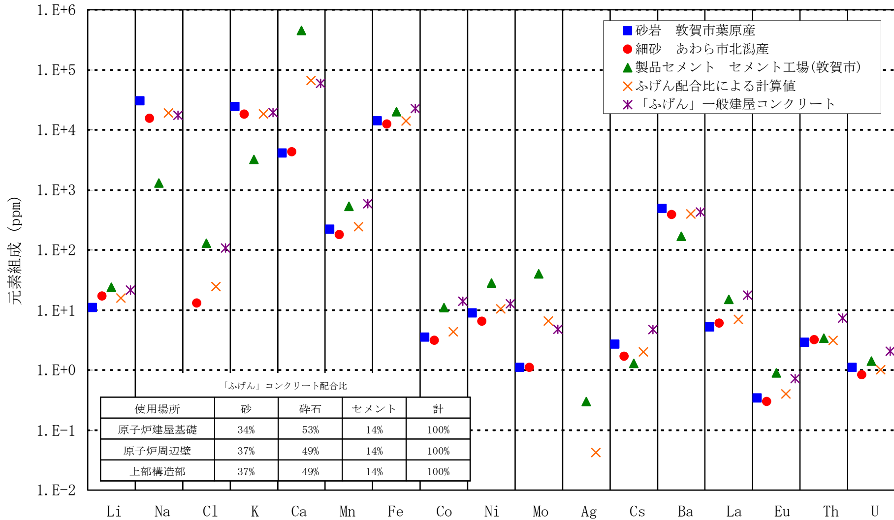
Fig.C 構造材の元素組成分析結果 (「ふげん」コンクリート配合比による計算値)
