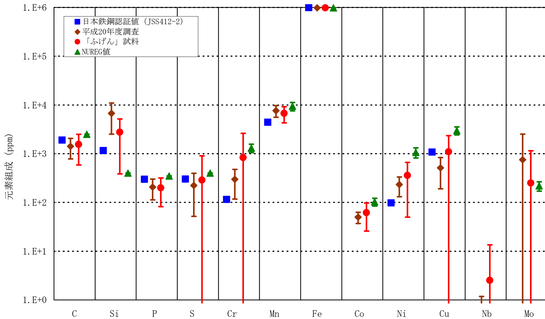
Fig. 5 構造材の元素組成の分析結果 (炭素鋼)
